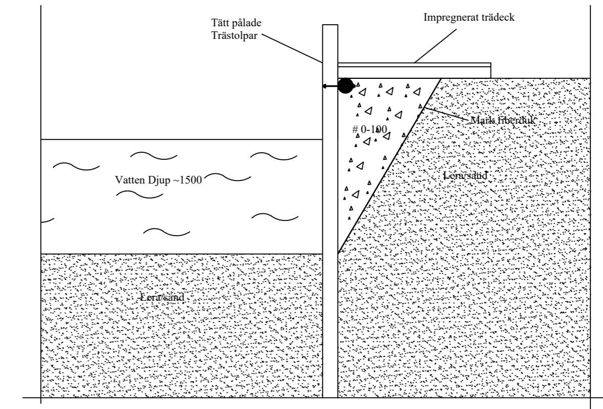
Pålade bryggans skärningsbild
