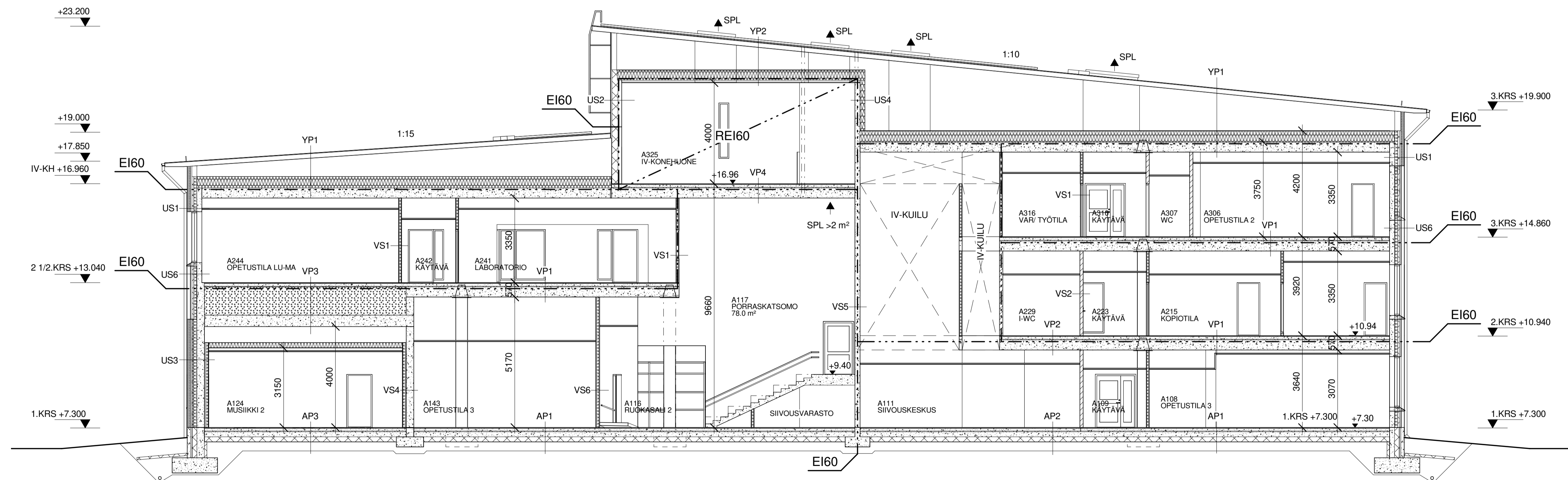
LEIKKAUS B-B
