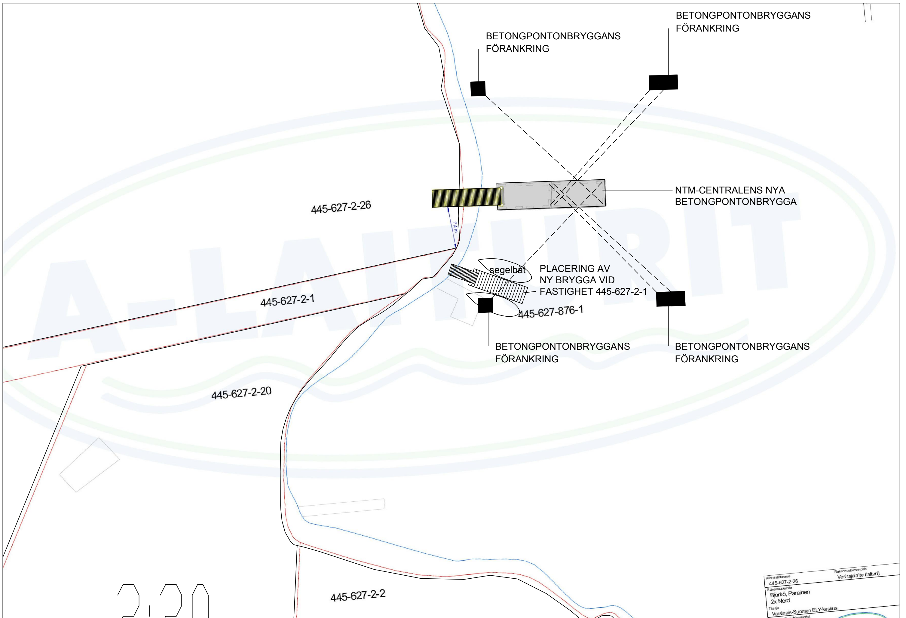
BJÖRKÖ NYA BETONGPONTONBRYGGA SKALA 1:400 A3 24.3.2021
