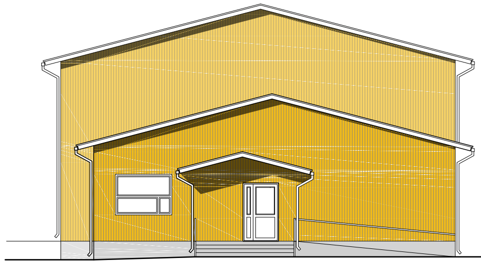
PÄÄTY ETELÄÄN
