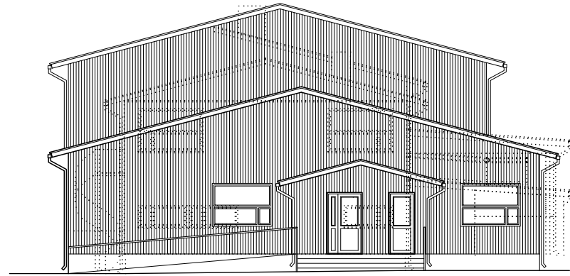
PÄÄTY ETELÄÄN
