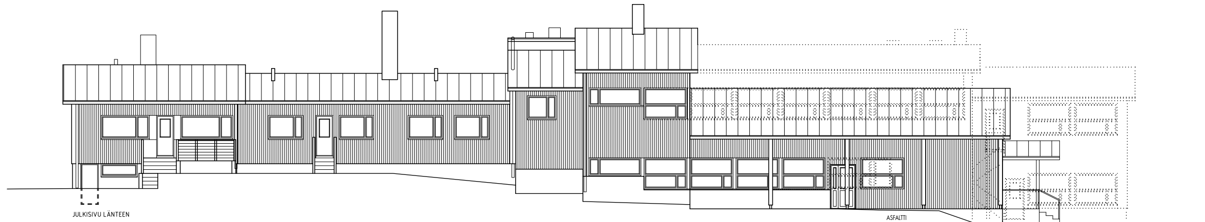
JULKISIVU LÄNTEEN
