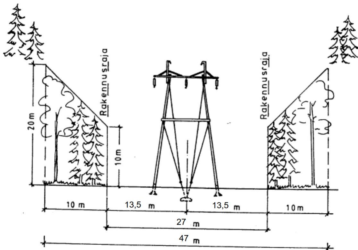
Kuva 1. Voimajohdon poikkileikkaus
