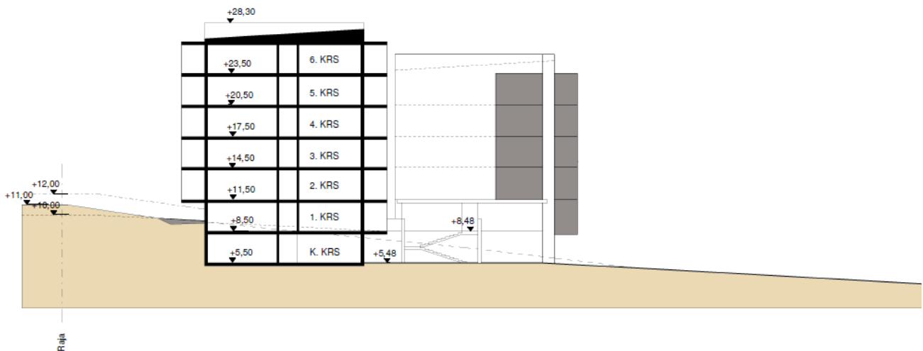
LEIKKAUS A-A
